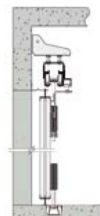
Posa oltre luce Installation to the wall Einbau auf der Wand
