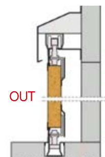
Sospeso con guida a terra Hanging with floor track Freitragend, mit Bodenführung
