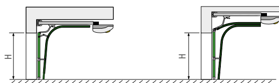
STA - Segmentna vrata sa jednostrukim vodjenjem
