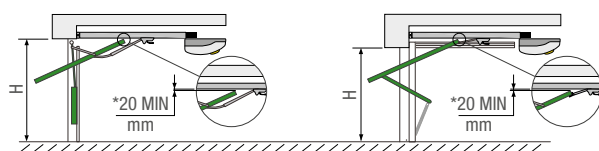
BC - Kiper vrata sa kontra tegom (con 001V201)
